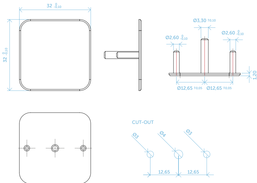
DIMENSÕES / MEDIDAS
